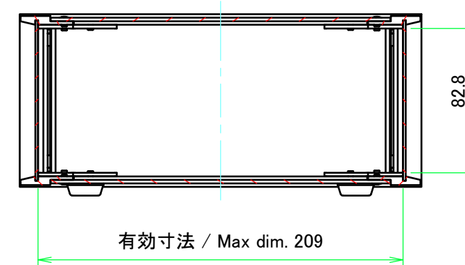
A-A ( 1 : 3 )
