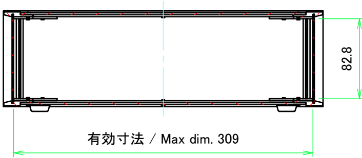
A-A ( 1 : 4 )
