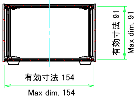
C-C ( 1 : 4 )
