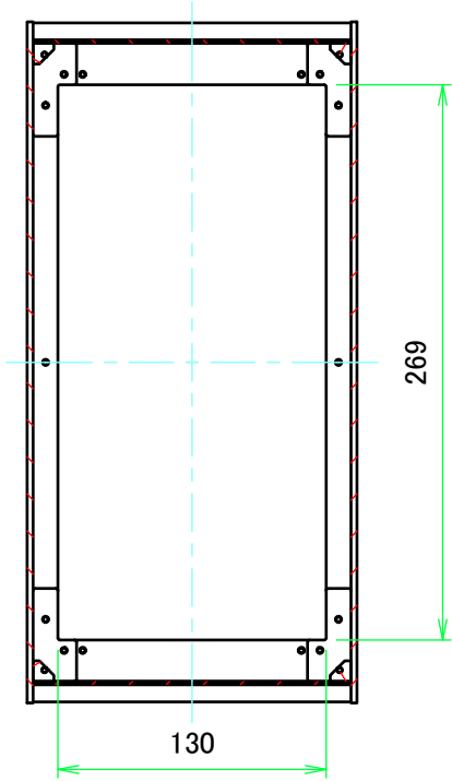
B-B ( 1 : 4 )
