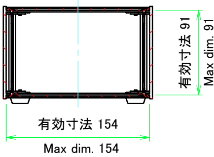
C-C ( 1 : 4 )
