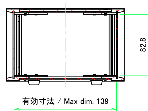
A-A (1:3)
