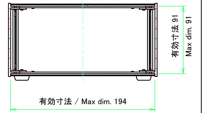
C-C ( 1 : 3 )
