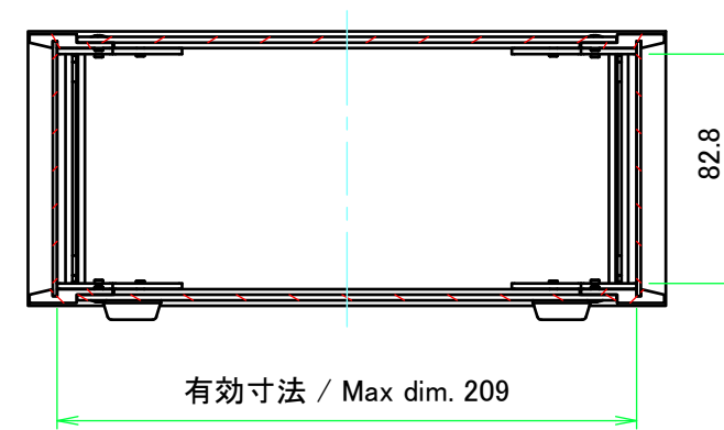
A-A ( 1 : 3 )
