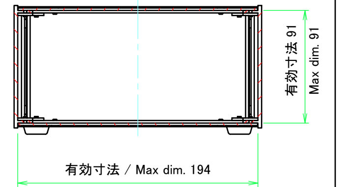
C-C ( 1 : 3 )
