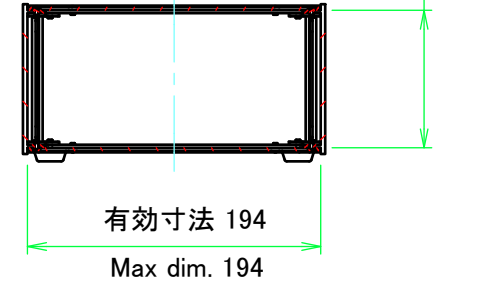
C-C ( 1 : 5 )
