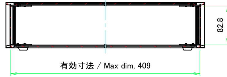
A-A ( 1 : 5 )
