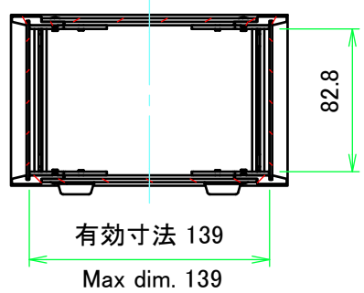
A-A ( 1 : 4 )
