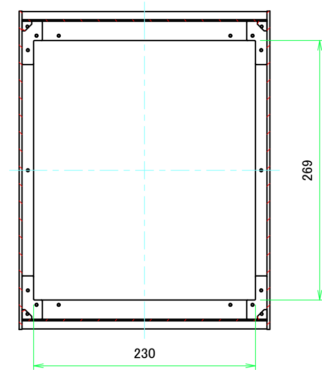
B-B ( 1 : 4 )
