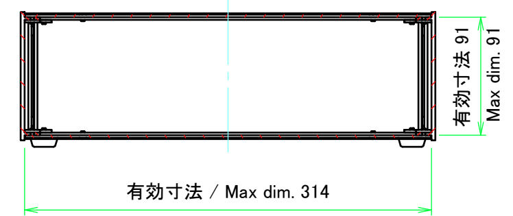
C-C ( 1 : 4 )
