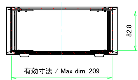
A-A ( 1 : 4 )
