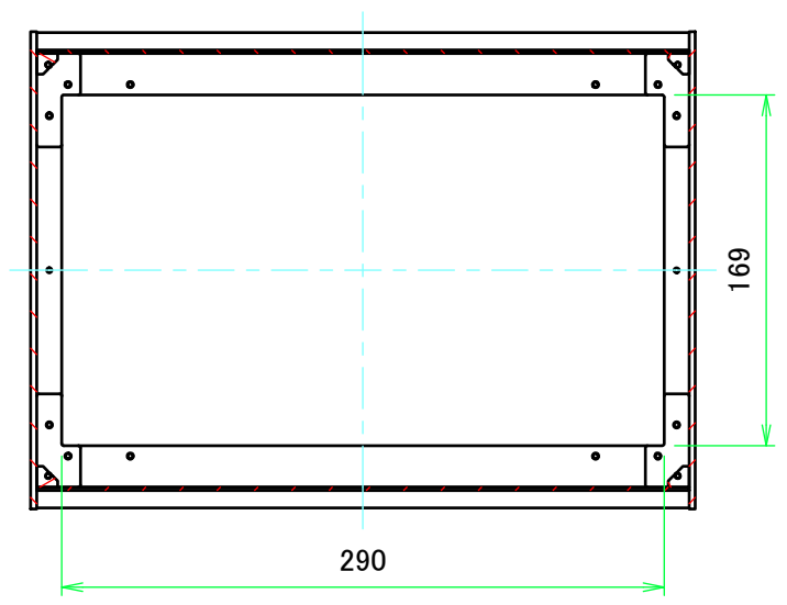
B-B ( 1 : 4 )
