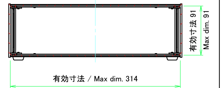
C-C ( 1 : 4 )
