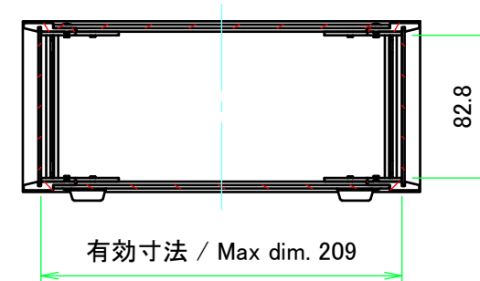
A-A ( 1 : 4 )
