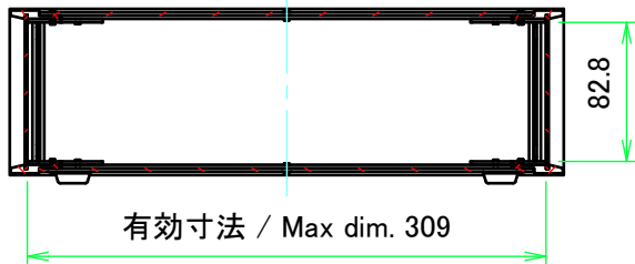
A-A (1:5)
