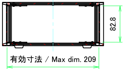
A-A (1:5)
