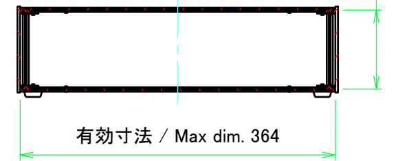
C-C ( 1 : 6 )
