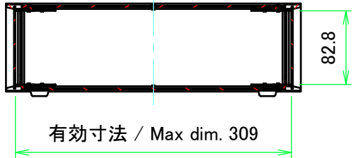
A-A (1:6)
