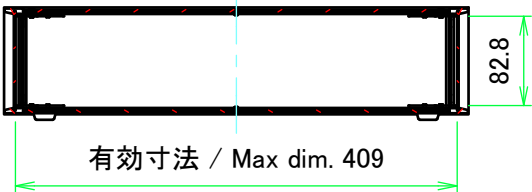
A-A ( 1 : 7 )
