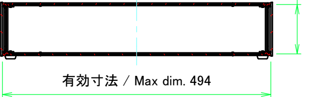
C-C ( 1 : 7 )
