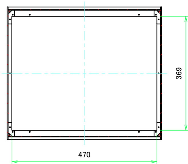
B-B ( 1 : 7 )
