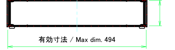
C-C ( 1 : 7 )
