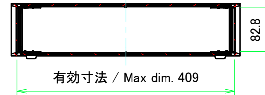
A-A ( 1 : 7 )
