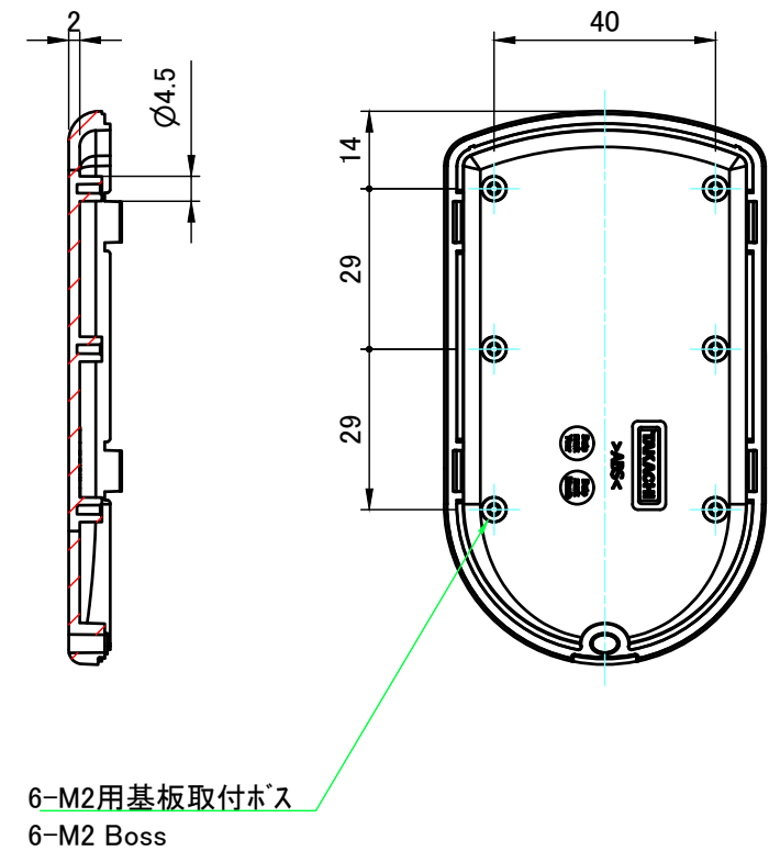
E-E ( 1 : 1.5 )
