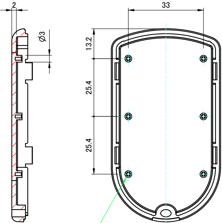
E-E ( 1 : 1 )
