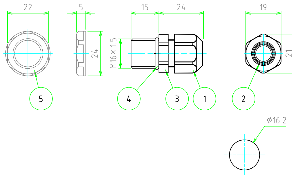
取付穴寸法 / Mounting hole dimensions
