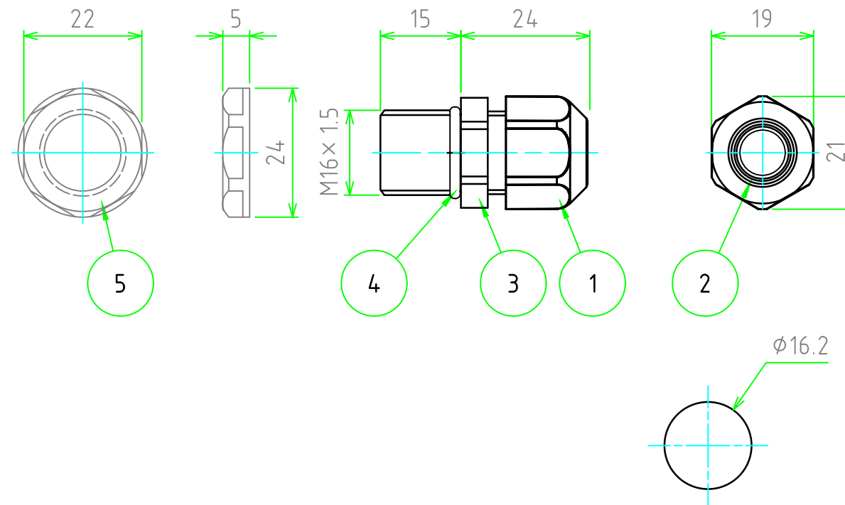
取付穴寸法 / Mounting hole dimensions
