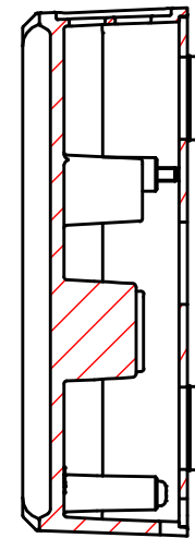
B-B ( 1:1.5 )
