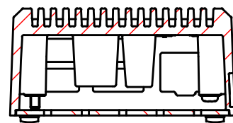
A-A ( 1:1.5 )
