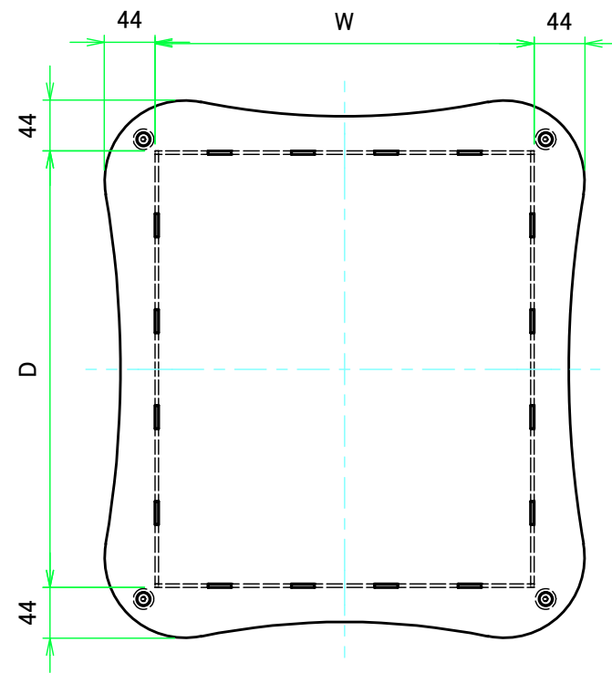
上カバー / Top cover
