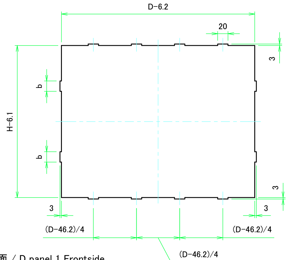
Dパネル1表面 / D panel 1 Frontside
