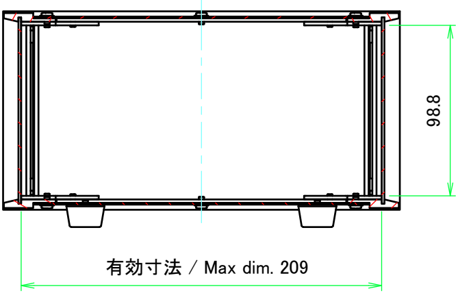
A-A ( 1 : 3 )
