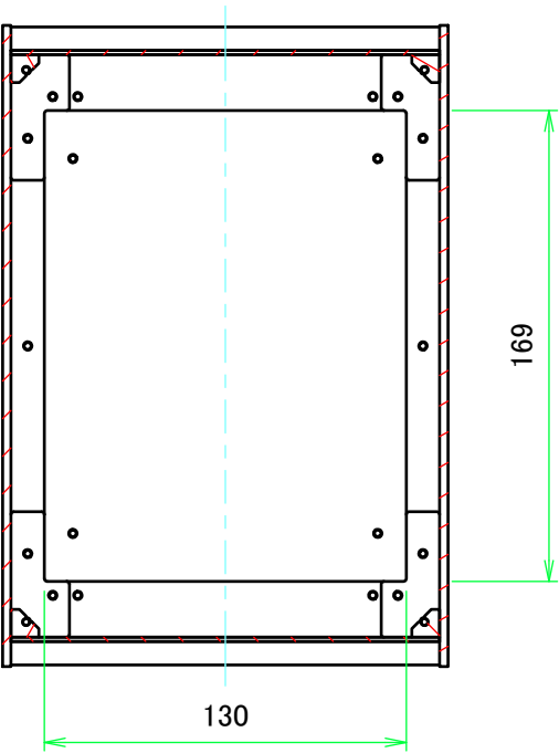
B-B ( 1 : 3 )
