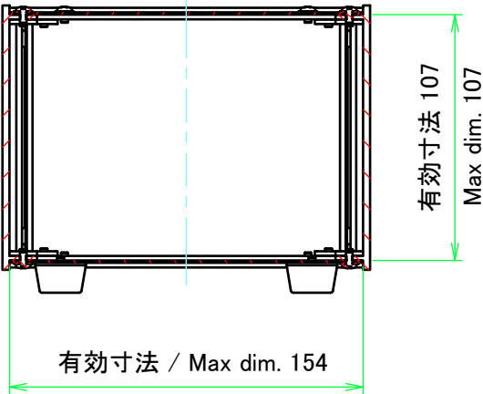
C-C ( 1 : 3 )
