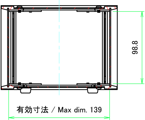
A-A (1:3)
