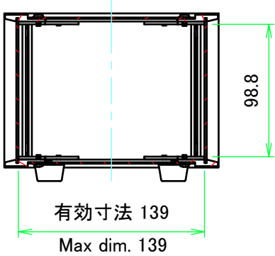
A-A ( 1 : 4 )
