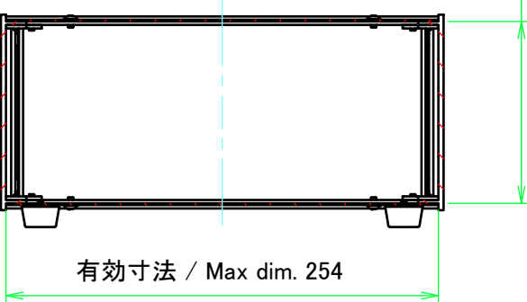
C-C ( 1 : 4 )
