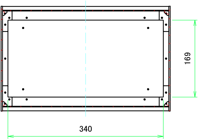
B-B ( 1 : 5 )
