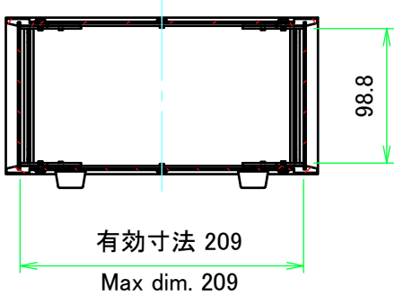
A-A ( 1 : 5 )
