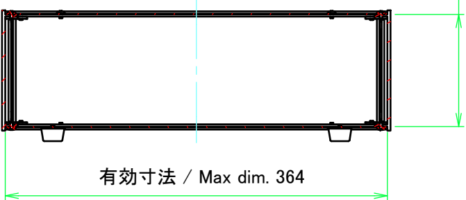
C-C ( 1 : 5 )
