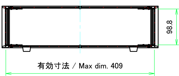
A-A ( 1 : 6 )
