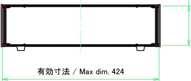
C-C ( 1 : 6 )
