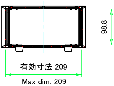
A-A ( 1 : 6 )
