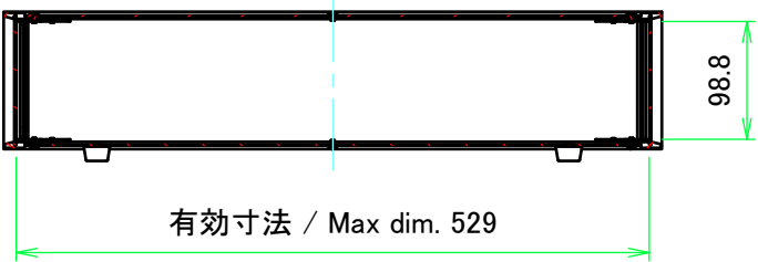
A-A ( 1 : 7 )
