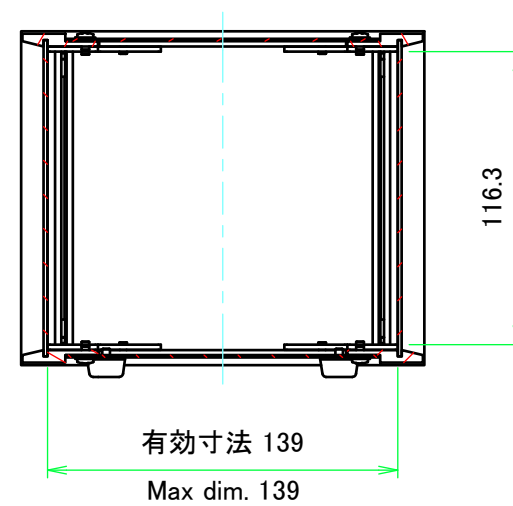
A-A (1:3)
