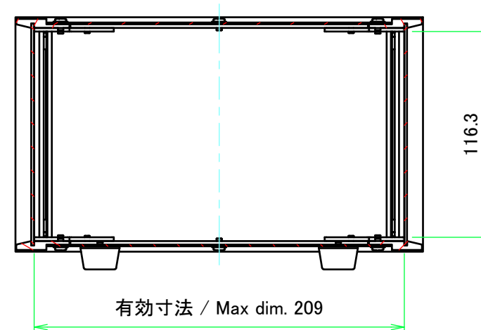
A-A (1:3)
