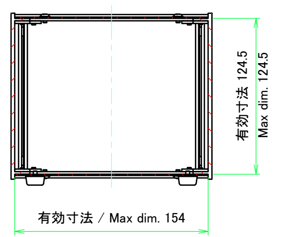
C-C ( 1 : 3 )
