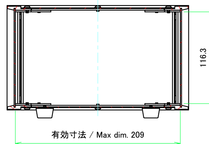
A-A (1:3)
