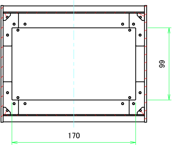
B-B ( 1 : 3 )
