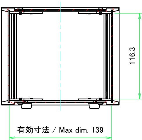
A-A ( 1 : 3 )
