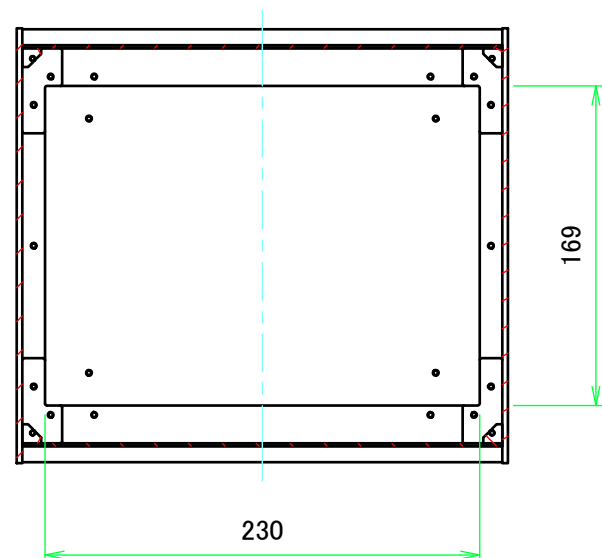
B-B ( 1 : 4 )
