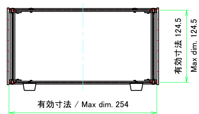
C-C ( 1 : 4 )
