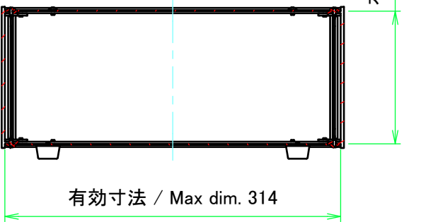
C-C ( 1 : 5 )
