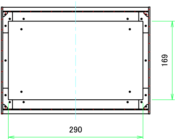
B-B ( 1 : 5 )
