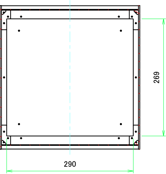
B-B ( 1 : 5 )
