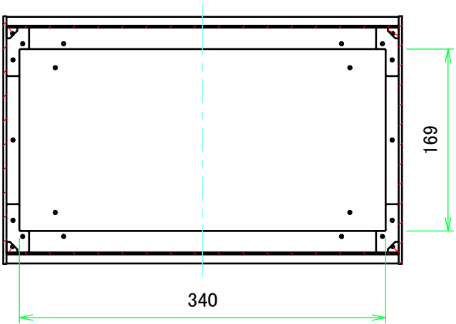
B-B ( 1 : 5 )
