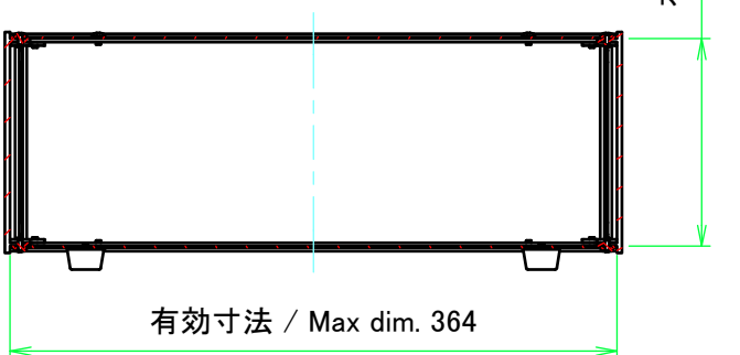
C-C ( 1 : 5 )
