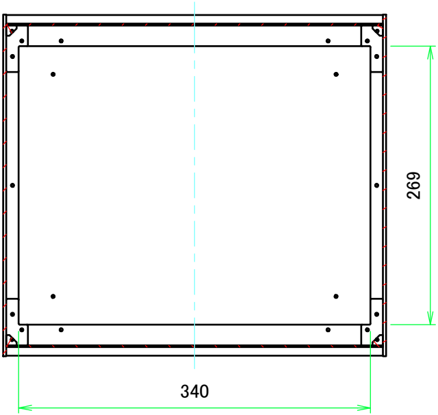
B-B ( 1 : 5 )
