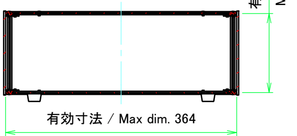
C-C ( 1 : 6 )
