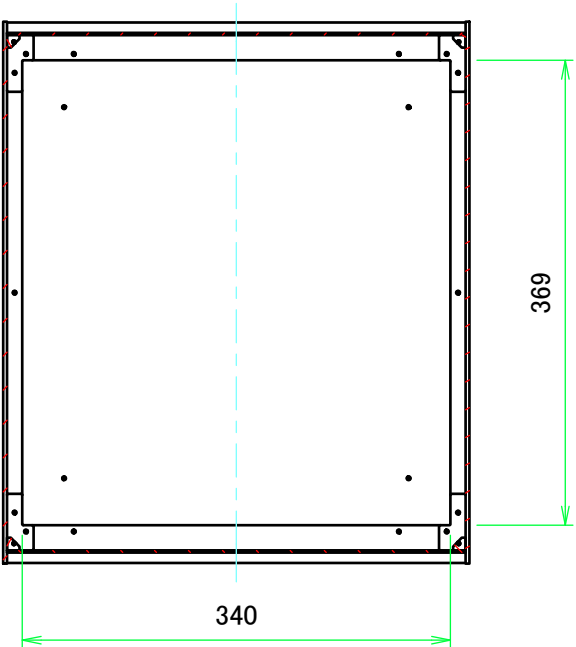
B-B ( 1 : 6 )
