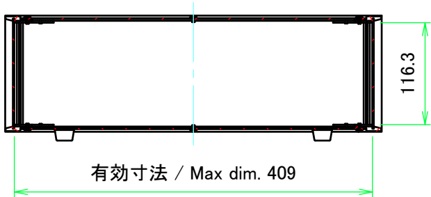
A-A ( 1 : 6 )
