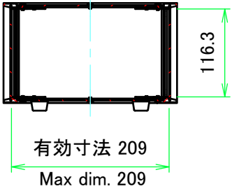
A-A ( 1 : 7 )
