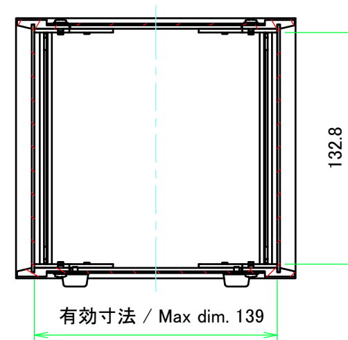
A-A (1:3)
