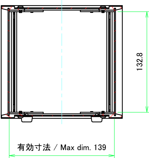
A-A ( 1 : 3 )
