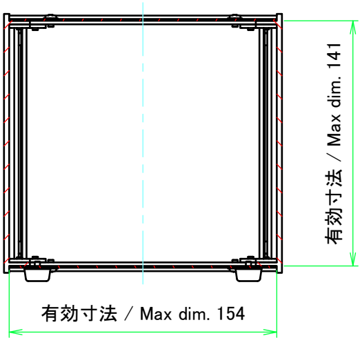
C-C ( 1 : 3 )
