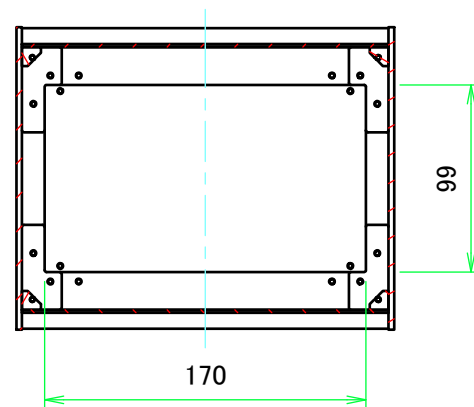
B-B ( 1 : 4 )
