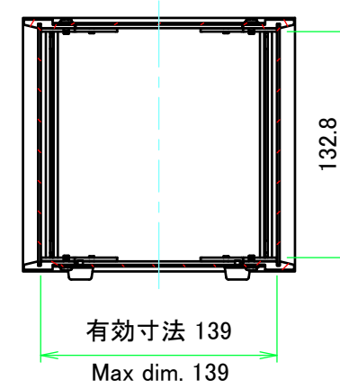
A-A ( 1 : 4 )
