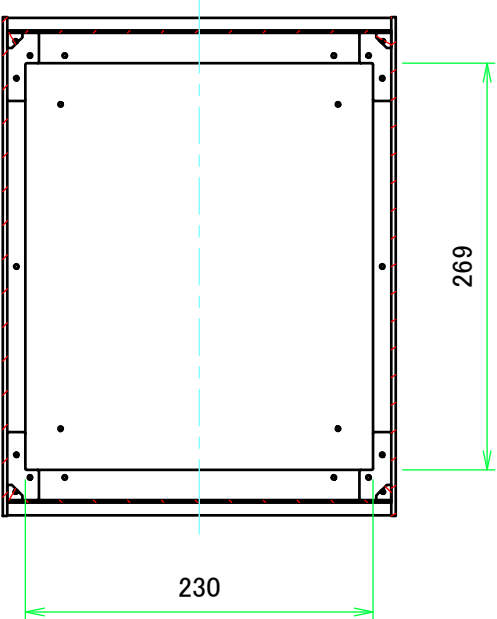
B-B ( 1 : 5 )
