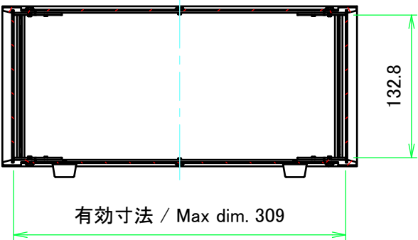
A-A ( 1 : 5 )
