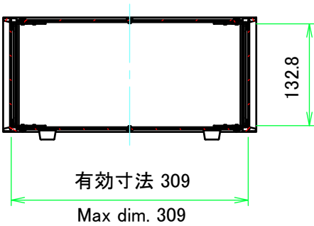
A-A ( 1 : 7 )
