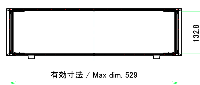
A-A (1:7)
