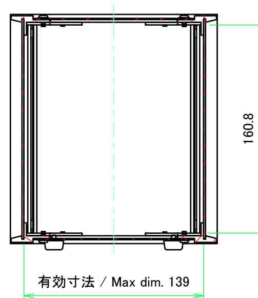
A-A (1:3)
