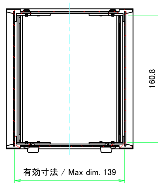
A-A (1:3)
